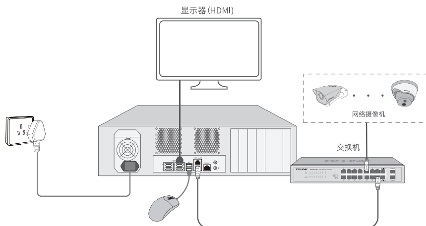
图3-4 NVR连接示意图
