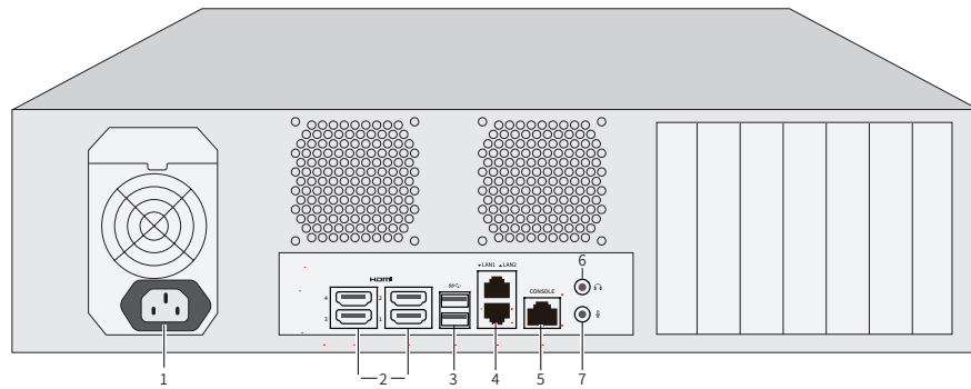
图1-3 TL-NVR8163-256S后面板示意图
