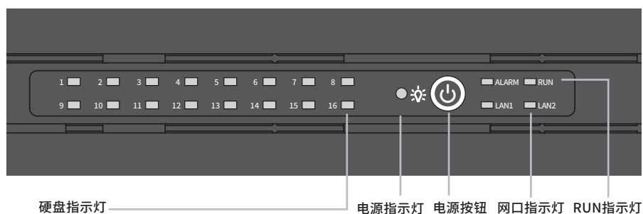
图1-2 前面板按钮与指示灯
