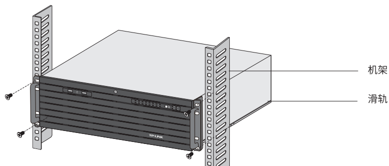
图2-2 机架安装示意图
