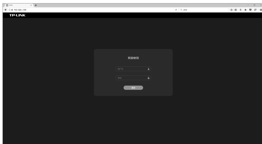
图5-2 登录界面
