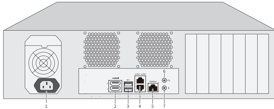
图1-4 TL-NVR8162-128S后面板示意图
