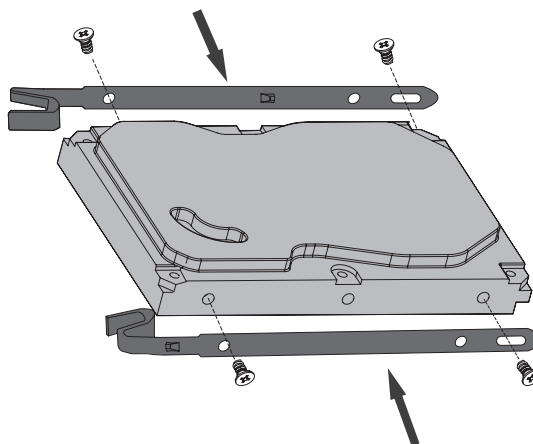
图3-2 安装硬盘支架
