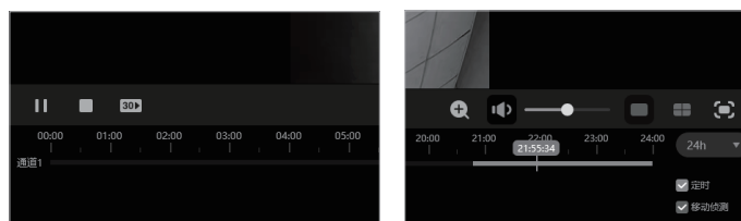
图5-5 操作栏
