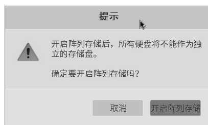
图4-5 确认风险
