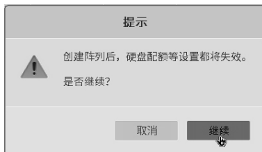
图4-7 确认创建
