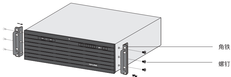
图2-1 角铁安装示意图
